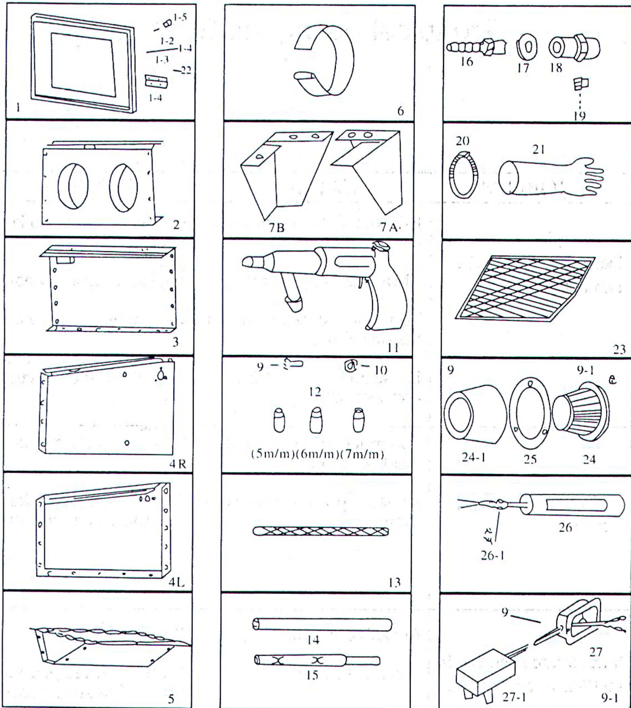
Abb. 7: Rozpadové schéma
